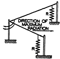
V antenna.
